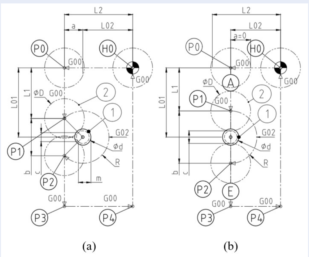
Hình 5: Sơ đồ xác định quan hệ hình học các thông số. (a) Góc chắn cung cắt AE > 180 (b) Góc chắn cung cắt AE = 180
