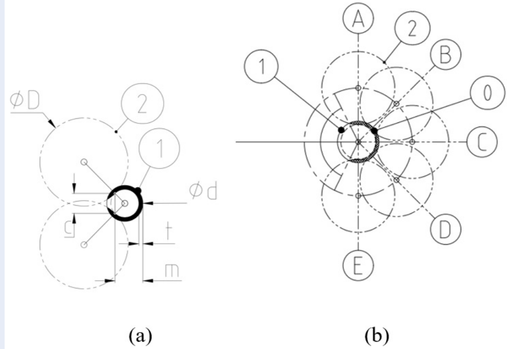
Hình 4: Sơ đồ gia công của vỏ cứng. (a) Các thông số đo trên sản phẩm. (b) Các các vị trí gia công.
