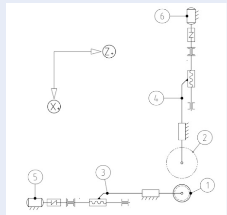
Hình 6: Sơ đồ tổ hợp truyền động 2 trục
