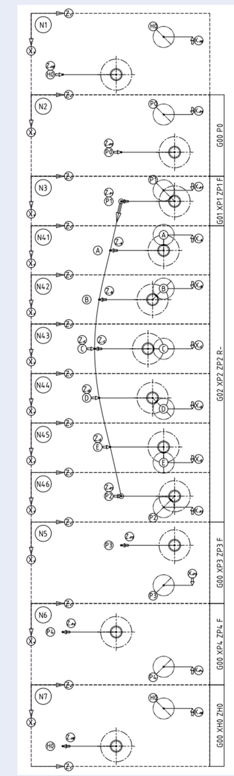
Hình 8: Sơ đồ tổ hợp động học 2 trục
