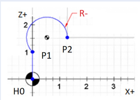
Hình 7: Các thông số bộ nội suy cung tròn G02.
