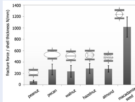
Hình 3: Lực phá hủy vỏ cứng của các loại hạt theo bề dày vỏ 1 .
