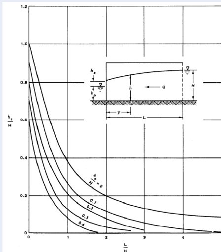
Hình 7: Biểu đồ tra độ chênh lệch h_s giữa mặt thoáng tự do và mực nước trong tầng chứa 1
