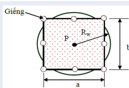
Hình 13: Bán kính ảnh hưởng của giếng lớn
