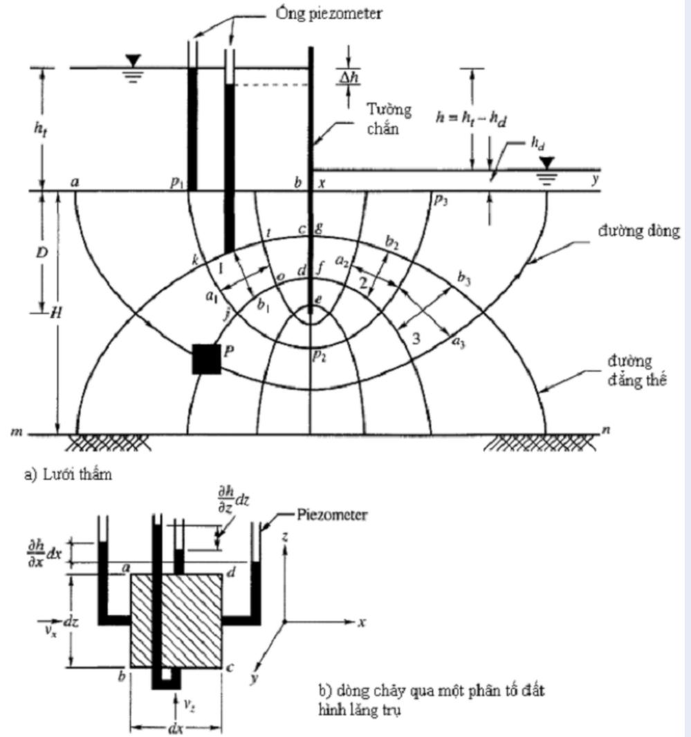
Hình 11: Dòng chảy qua một tầng đất đồng nhất
