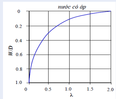
Hình 5: Biểu đồ quan hệ giữa tỉ số W/D và hệ số \lambda
