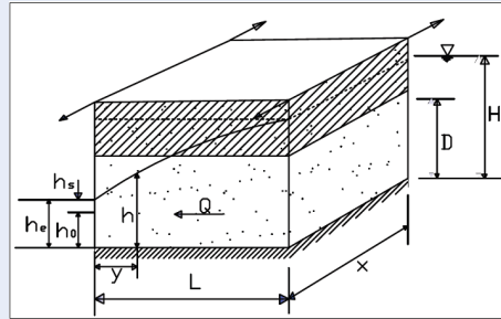
Hình 9: Hào hoàn chỉnh có nguồn cấp từ 1 phía trong tầng nước có áp
