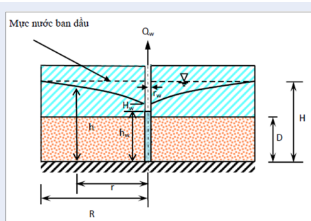
Hình 10: Giếng đơn có nguồn cấp từ hai phía
